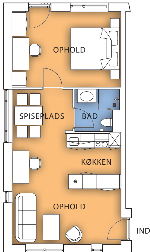
LEJLIGHED TYPE A Spejlvendt som TYPE AS mål 1:100 areal 61,8 m 2
