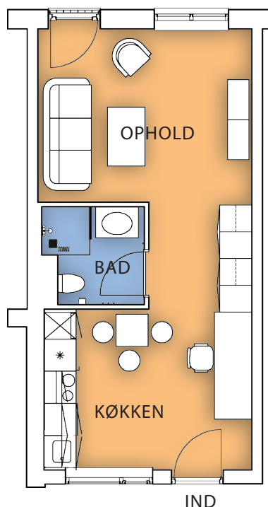
LEJLIGHED TYPE C Spejlvendt som TYPE CS mål 1:100 areal 43,5 m 2
